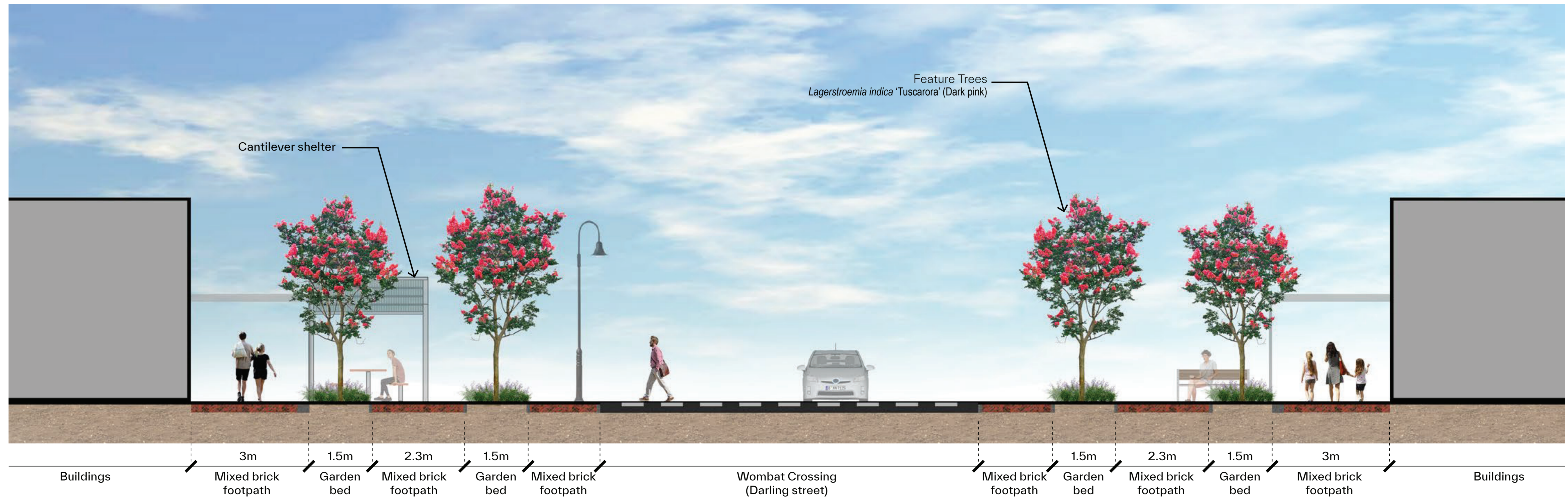
SECTION B-B 1:100 @A3
