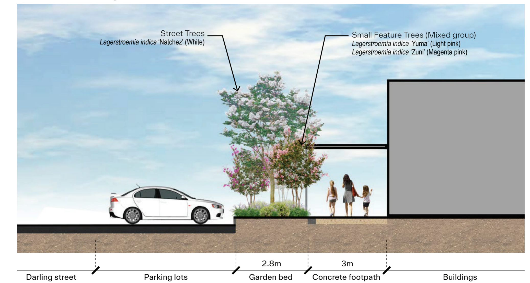
SECTION A-A 1:100 @A3
