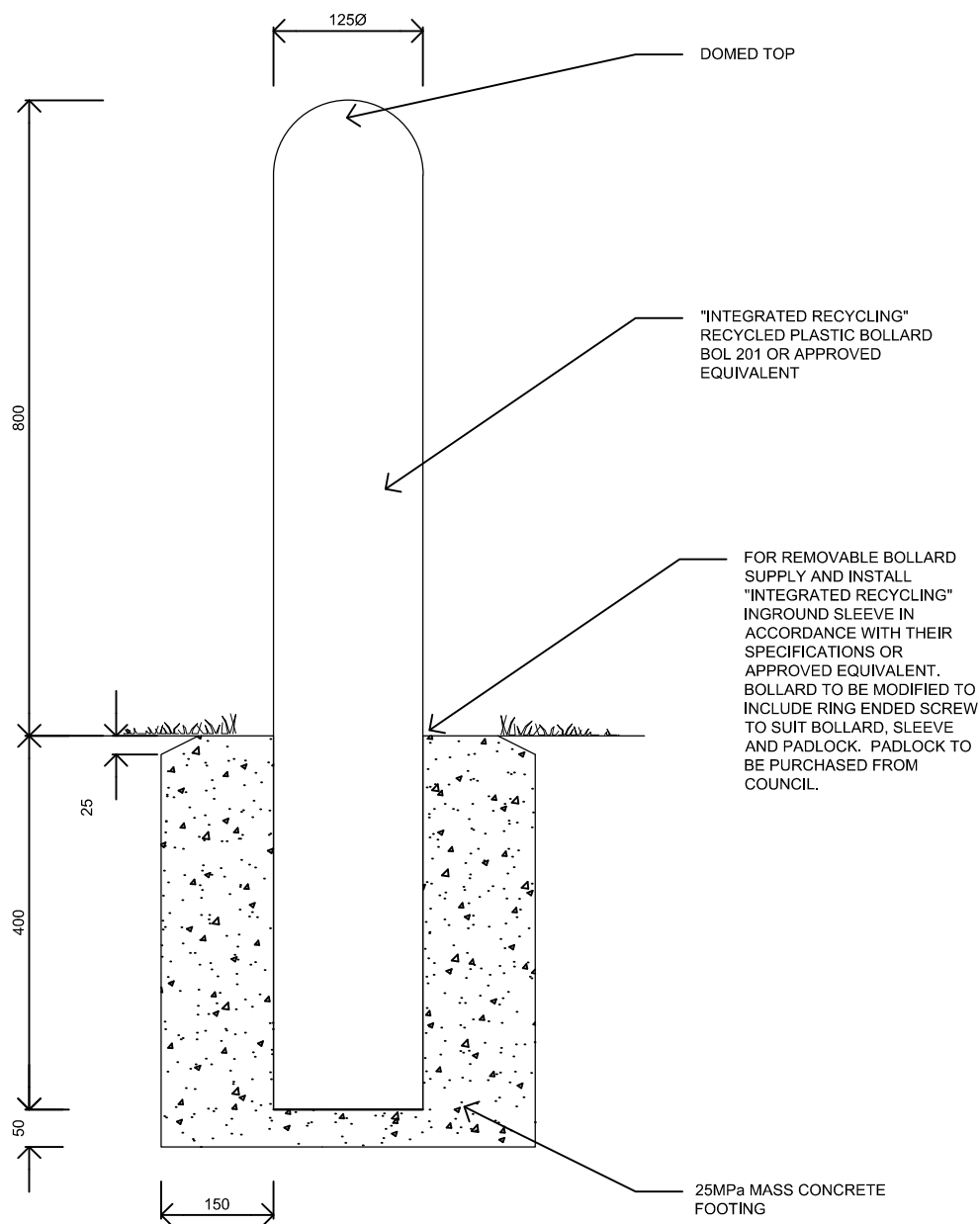
ELEVATION
