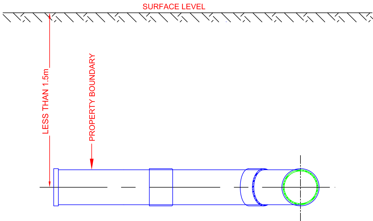
ELEVATION
