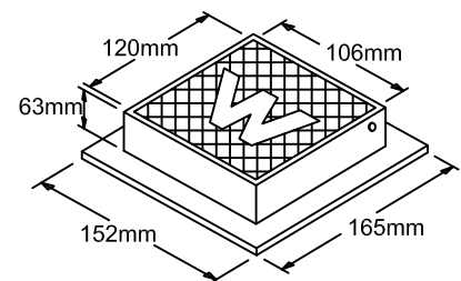
PATH BOX DETAIL (N.S.W.)
